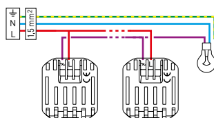
2 automatische schakelaars
